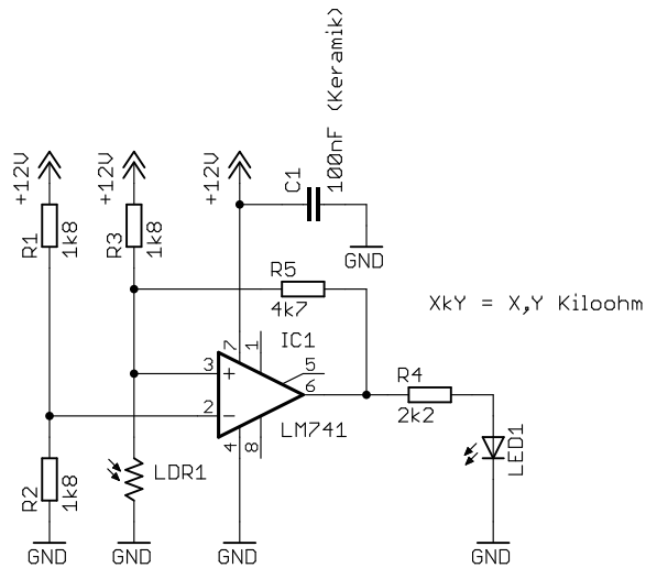
Dämmerungsschalter mit Hysterese (Schmitt-Trigger)
